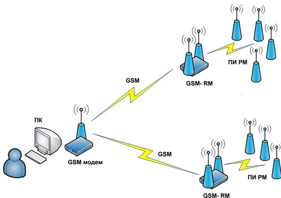
Рис. 10 – Структурная схема GSM/PM сети
