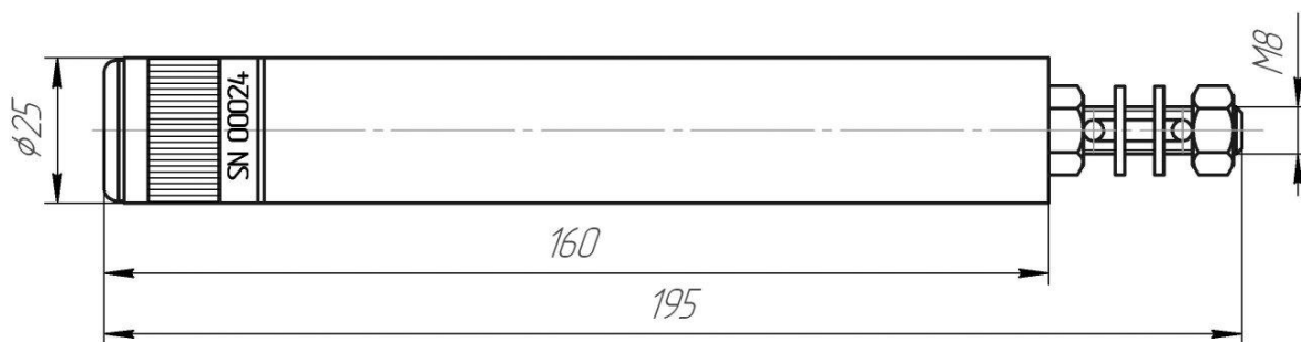
Рис. 4 – Логгер ЛЦД-1/100
