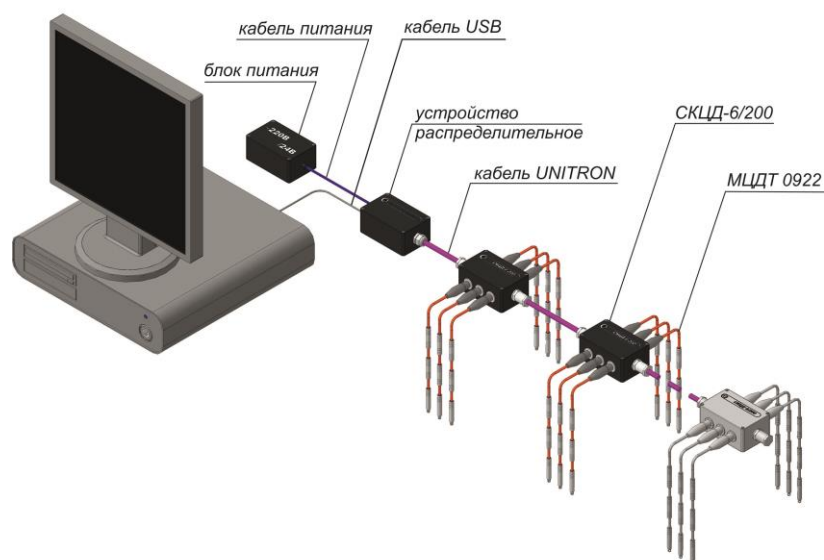
Рис. 2 – Схема реализации СТМ ПО
